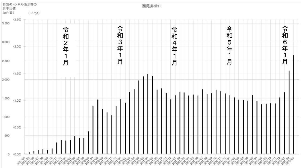
図 参 2-1 西尾非常口工事施工ヤードのトンネル湧水等 注1 の状況 注2
